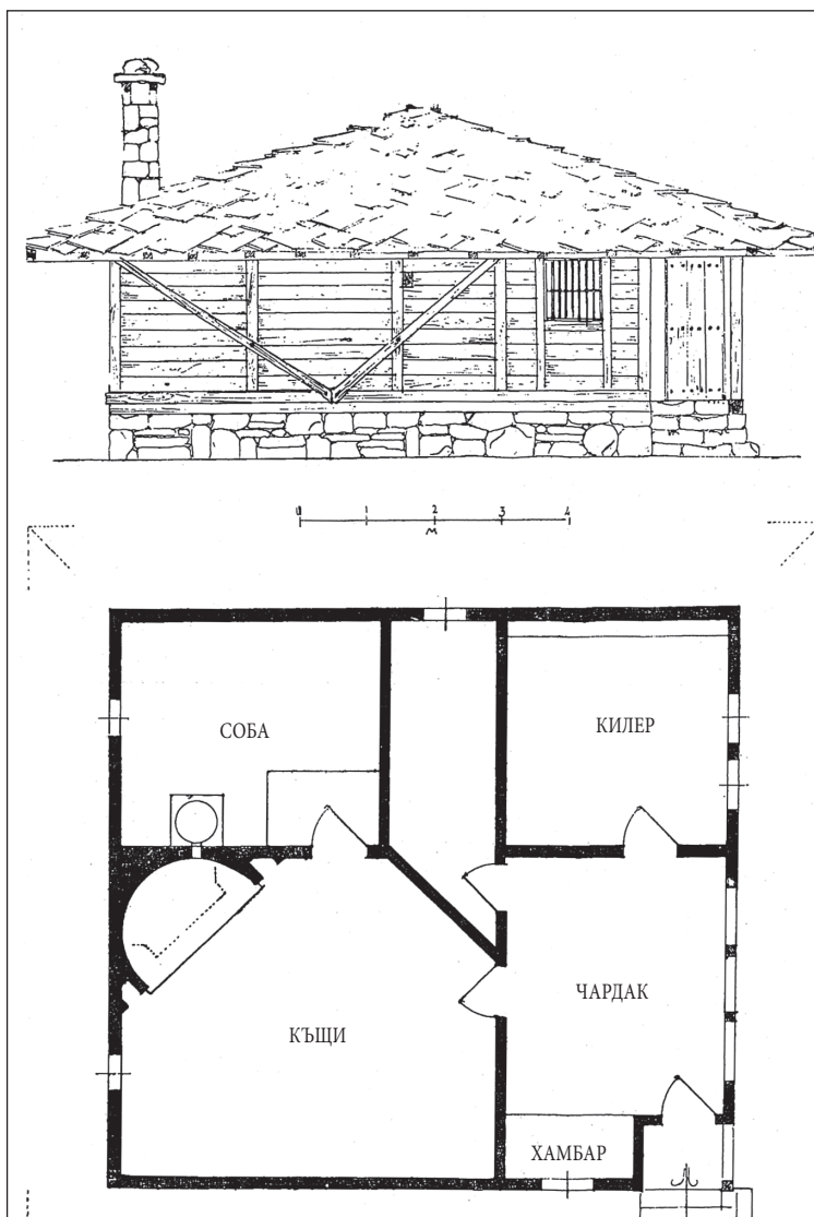
Разпределение и фасада на къщата на Лазар Матев в с. Стайновци, Тревненско, строена в началото на XVIII в.
